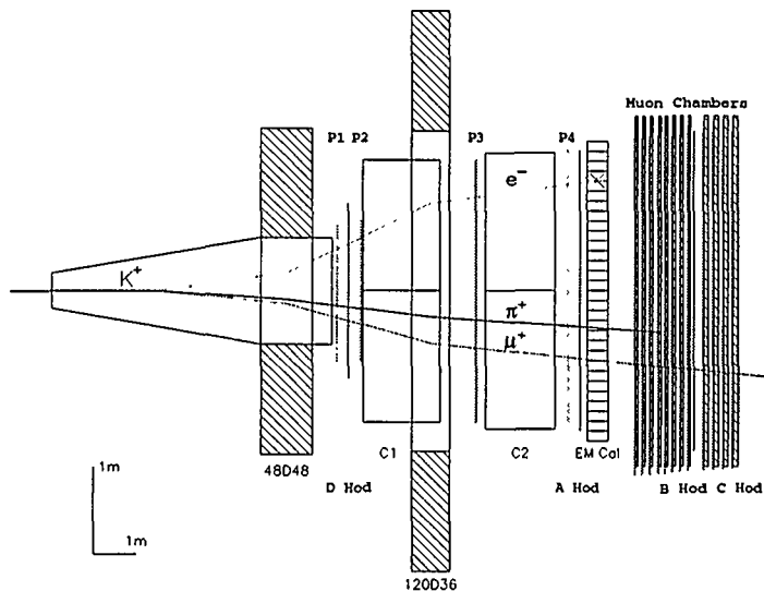
E865, Plan Diagram, K^+ \rightarrow \pi^+ \mu^+ e^-
